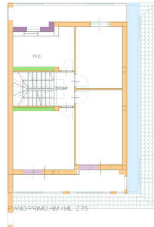
PIANO PRIMO
