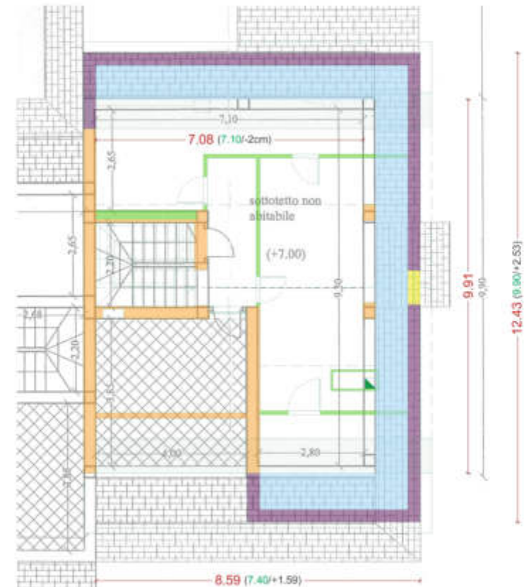
PIANO SECONDO (SOTTOTETTO)
