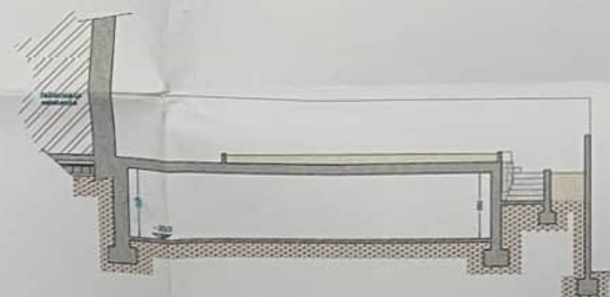
sezione Y-Y
