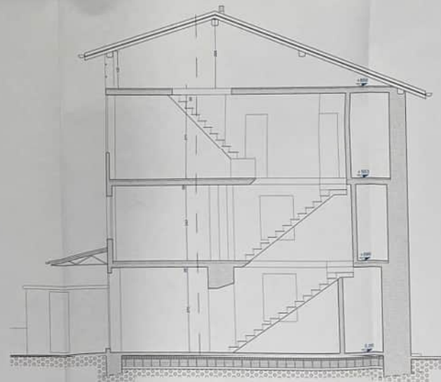
sezione A-A
