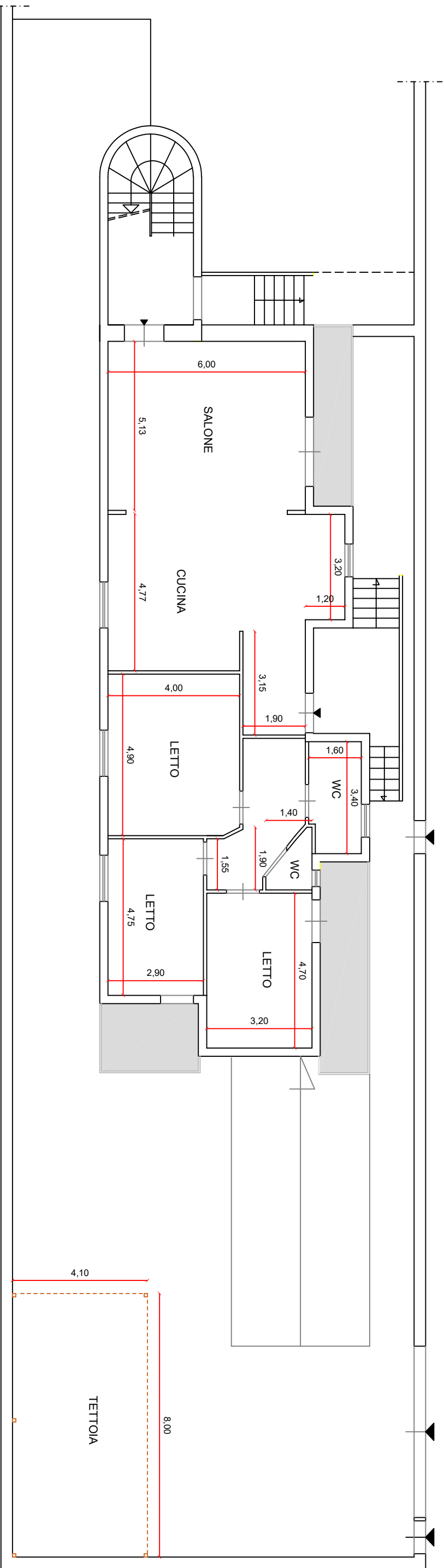
PIANTA PIANO TERRA
