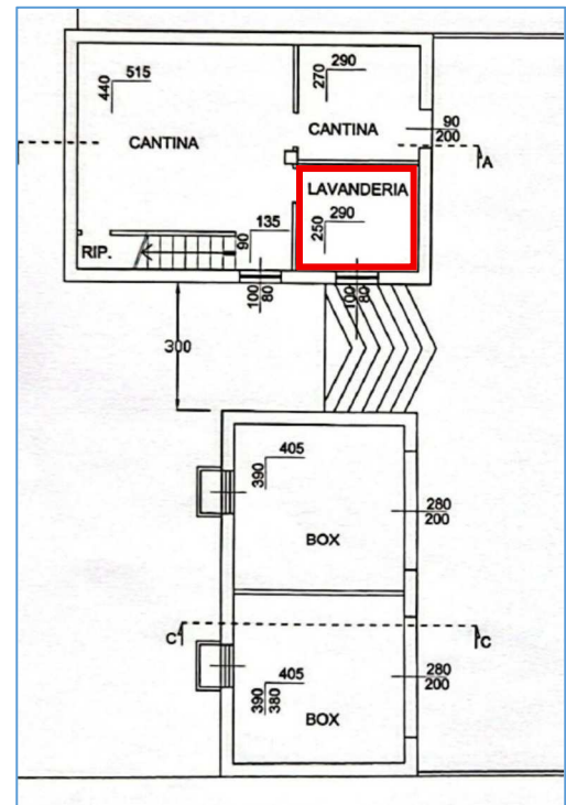
Stralcio tavola progettuale piano primo sottostrada
